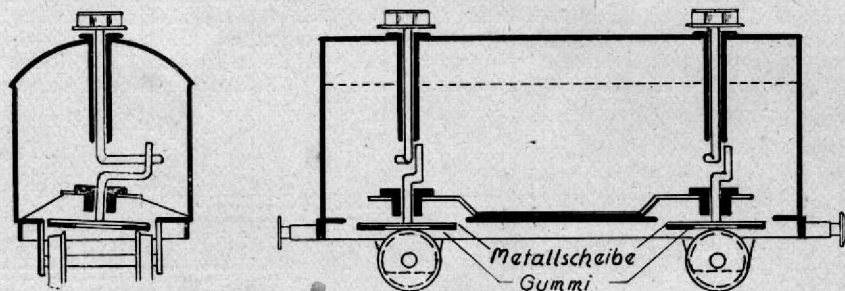
Abb. 2: Antriebsschema für Flettnerlüfter.
