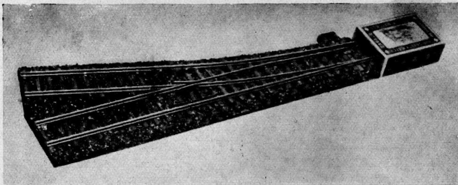
Abb. 1. Fertige Rechtsweiche mit eingebautem Antrieb. Weichenlaterne weggelassen. Der Streichholz-„Prellbock“ dient lediglich zur Veranschaulichung des Gleisbettungskörpers.
