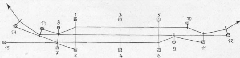
Abb. 5: Verdrahtung des Bahnhofs „Holzingen“.
