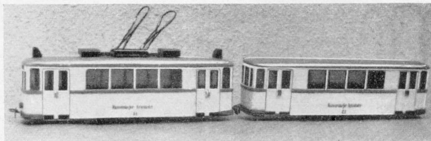
Meterspur-Straßenbahnzug der „Rumxendorfer Kreisbahn“. Maßstab 1:45, Spurbreite 24 mm, aus Aluminiumblech 0,35 mm und Kunststoff, gebaut von Herrn Jaeschke.
