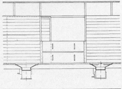
Schnitt C — D
